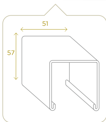
Boitier métallique Head rail
