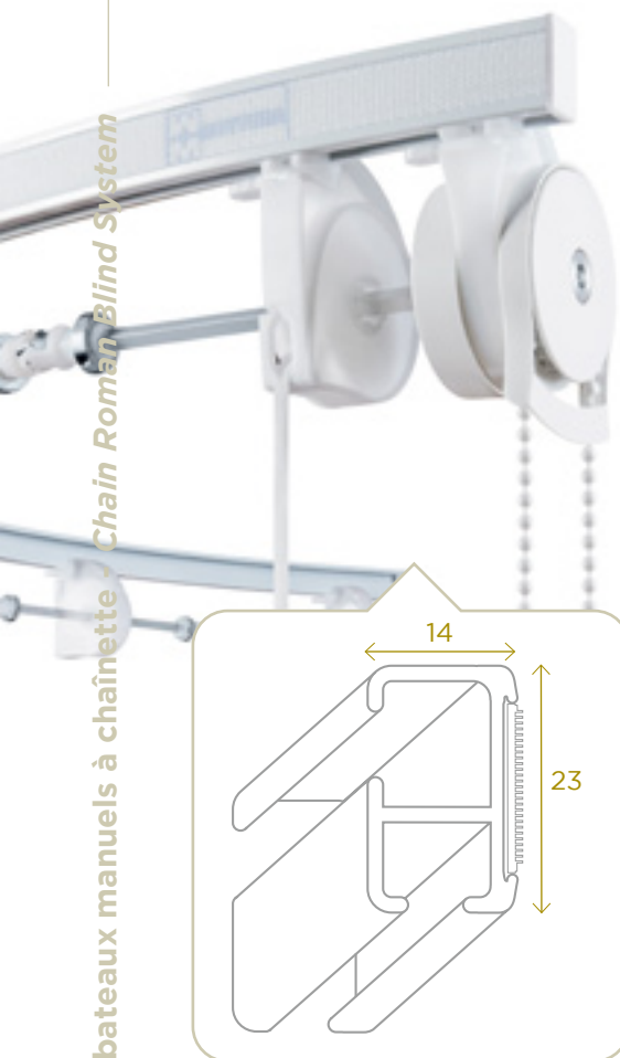
Profil 14x23 14x23 profile
