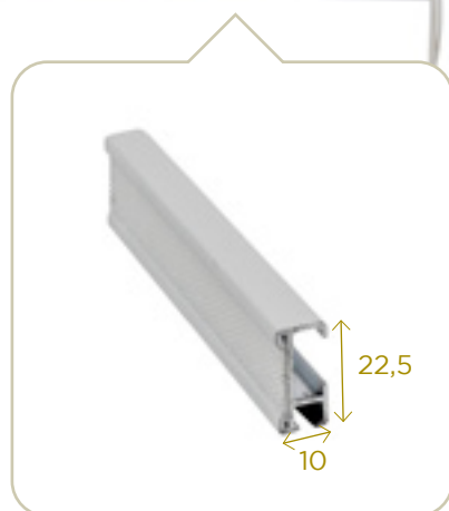
Profil SG 2116 SG 2116 profile
