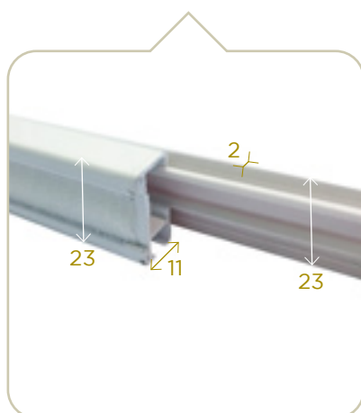
Profil + profil adhésif Profile + adhesive profile
