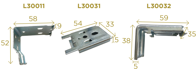
Supports pour façade et coffre Fascia and cassette brackets
