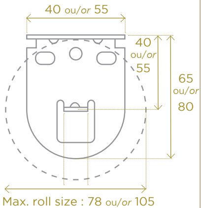
ENROULEMENT MAX MAX ROLL
