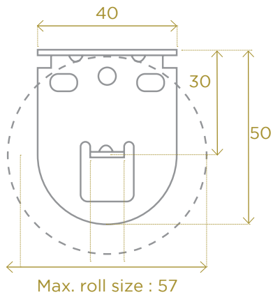
ENROULEMENT MAX MAX ROLL
