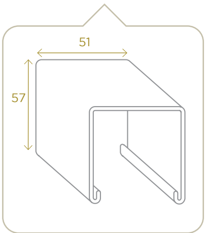
Boîtier métallique Head rail
