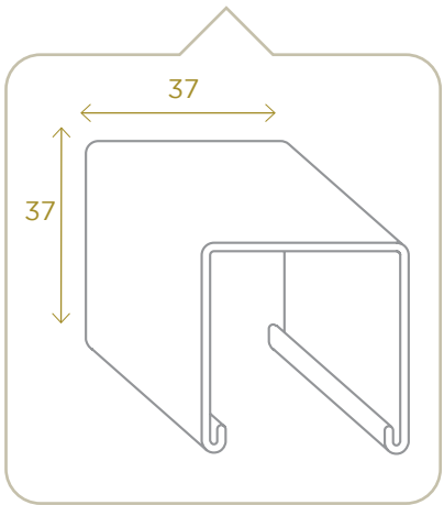
Boitier métallique Head rail
