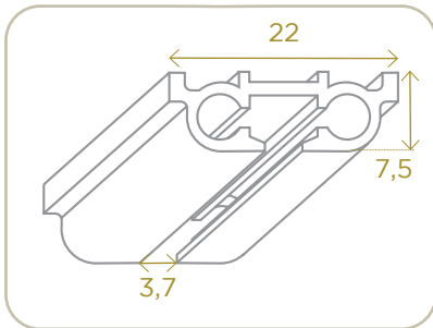
Schéma pour cotes uniquement Dimensions diagram (not to scale).
