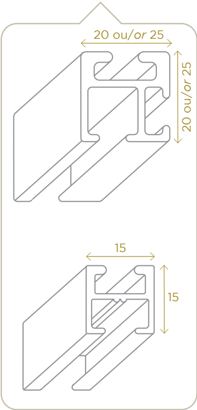
Profil (cote : 15x15/20X20/25x25) Profile (dimensions: 15x15/20X20/25x25)
