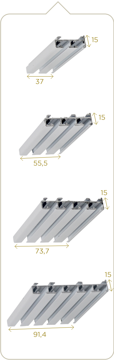
Profil de 2 à 5 rails Profile 2 to 5 channels
