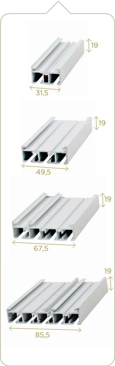
Profil SG 2700 SG 2700 profile
