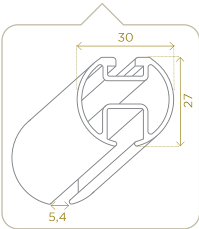
Profil SG 6130 SG 6130 track profile
