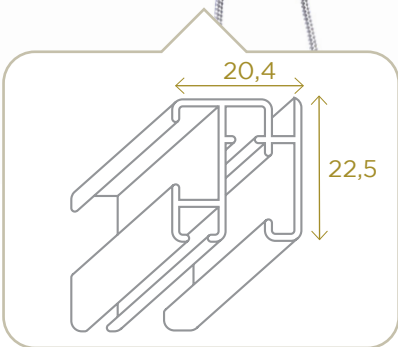
Schéma pour cotes uniquement Dimensions diagram (not to scale).
