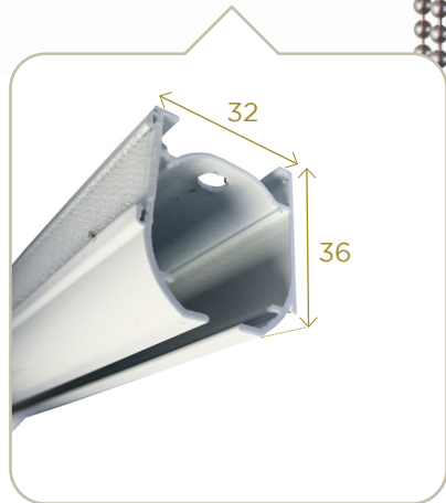
Profil 32x36 32x36 profile
